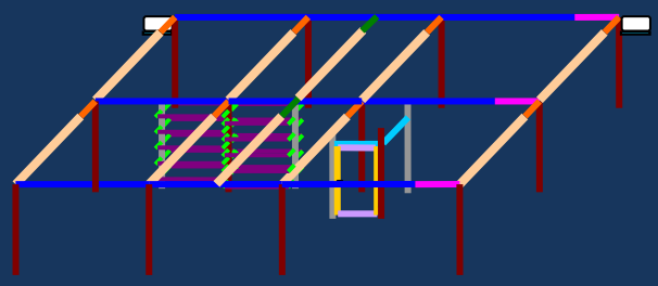
Stand "à géométrie variable", 2 configurations de montage possibles
