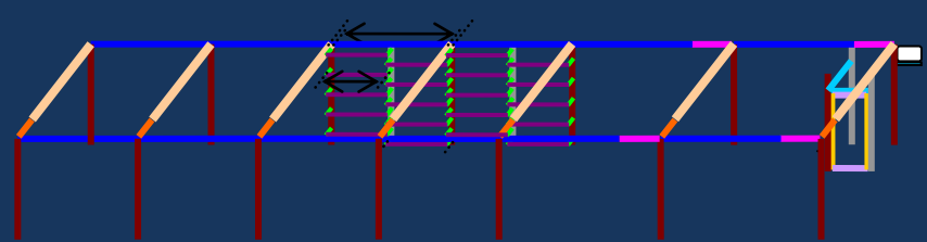
Stand "à géométrie variable", 2 configurations de montage possibles
